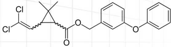
Permethrin
